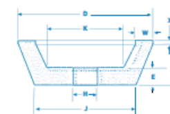
Tipo 11, Copa de cara afilada
