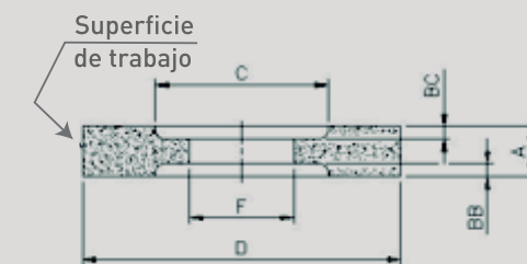
TIPO 7 - Perfil por dos lados
